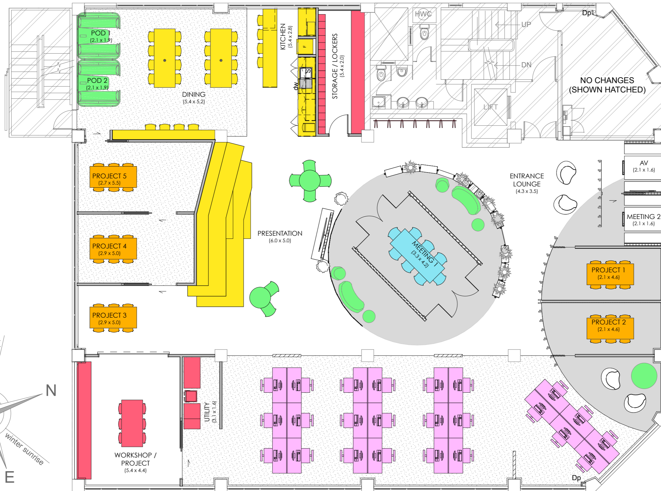
EMPATHY FIT OUT - Concept Plan 01 1:100
