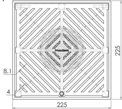
Top
